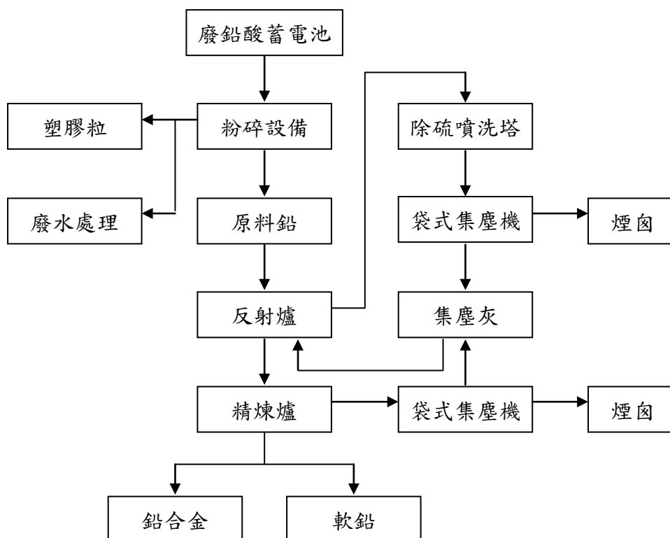
圖二：廢鉛酸蓄電池回收作業流程
